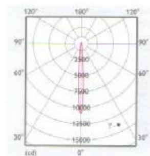
MASTERline ES 12V 30W 6dgr
